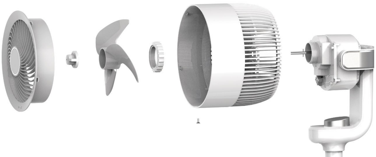
羽根やガードの分解イメージ
